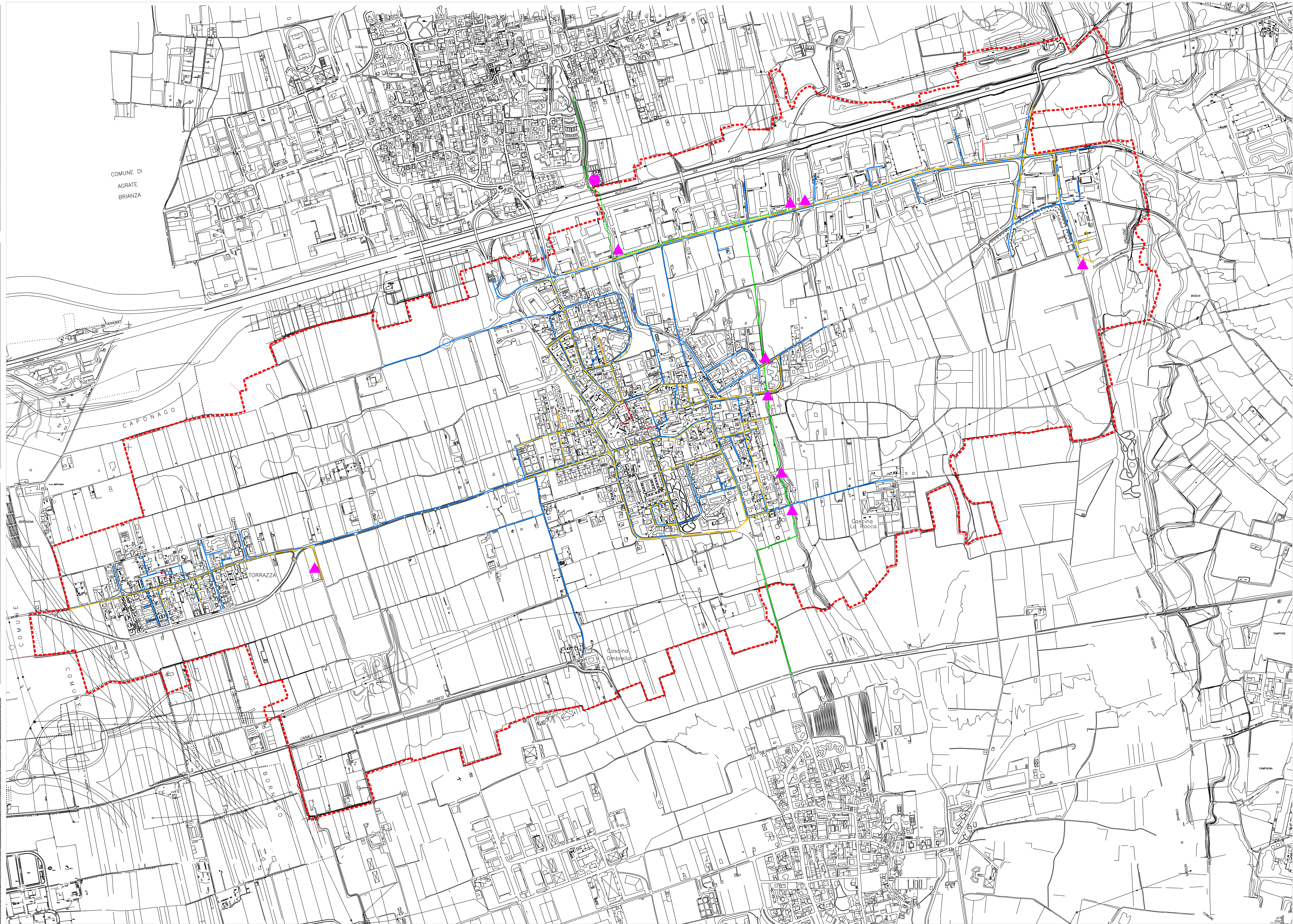
NODI DELL'IMPIANTO DI ACQUEDOTTO: STAZIONI DI SOLLEVAMENTO
